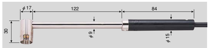
●SK-S308K 静止表面用 (L 型センサ、中温) -30~600℃ 先端部φ17×ℓ30mm コード1.1m付 No.8080-64 ¥15,000 (税込¥15,750) (センサ精度 クラス2)
