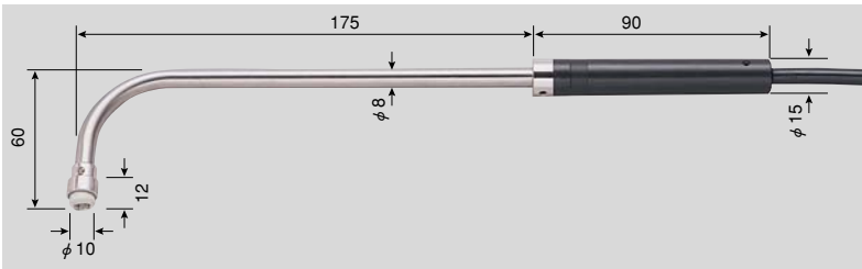
●SK-S303K 静止表面用 L 型 (中・高温用) 0~800℃ 先端部φ10×ℓ12mm コード1.1m付 No.8080-54 ¥13,000 (税込¥13,650) (センサ精度 クラス2)
