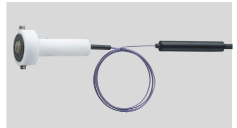
●SK-S403K 静止表面用 (マグネット型) 0~200℃ 先端部φ30×ℓ12mm 取っ手部φ15×ℓ50mm コード1.1m付 ¥19,500 (税込¥20,475) (センサ精度 クラス2)
