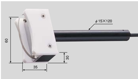
●SK-S401K 曲面表面用 (パイプ等) 0~250℃ 先端部30×35×60mm コード1.1m付 No.8080-70 ¥16,500 (税込¥17,325) (センサ精度 クラス2)
