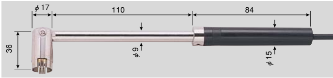
●SK-S305K 静止表面用 (90° 角度可変、中温) -30~500℃ 先端部φ17×ℓ36mm コード1.1m付 No.8080-58 ¥19,500 (税込¥20,475) (センサ精度 クラス2) (写真は90°に曲げた状態)
