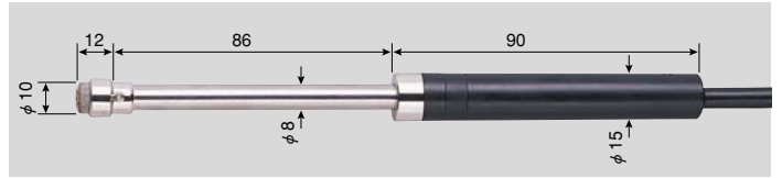
●SK-S306K 静止表面用 (低温) -30~250℃ 先端部φ10×ℓ12mm コード1.1m付 No.8080-60 ¥13,000 (税込¥13,650) (センサ精度 クラス2)
