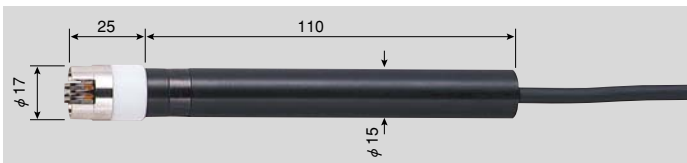
●SK-S307K 静止表面用 (一般計測、低温) -30~400℃ 先端部φ17×ℓ25mm コード1.1m付 No.8080-62 ¥13,000 (税込¥13,650) (センサ精度 クラス2)
